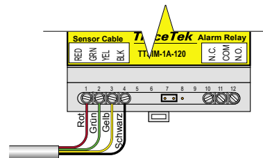
Abbildung 6. Anschluss der Sensorkabel
