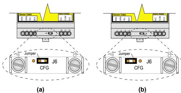
Abbildung 8. CFG Stecker Position zur Konfiguration (a) und normalen Betrieb (b)
