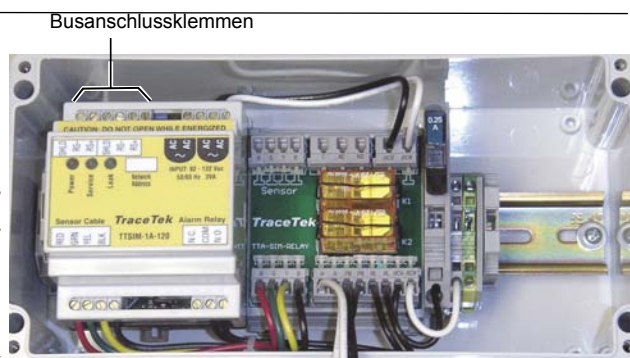
Abbildung 6. Busanschluss
