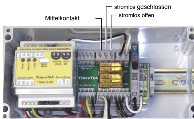
Abbildung 5. Relaisanschluss
